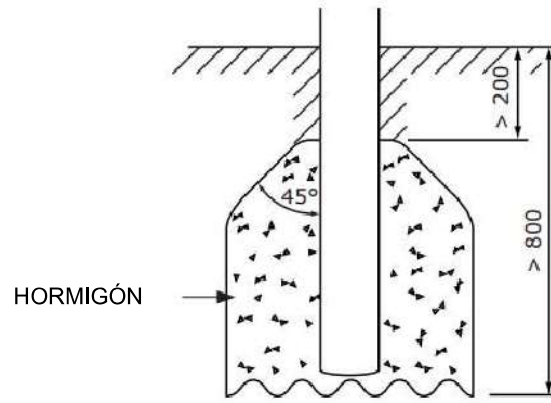
DETALLE CIMENTACIÓN
